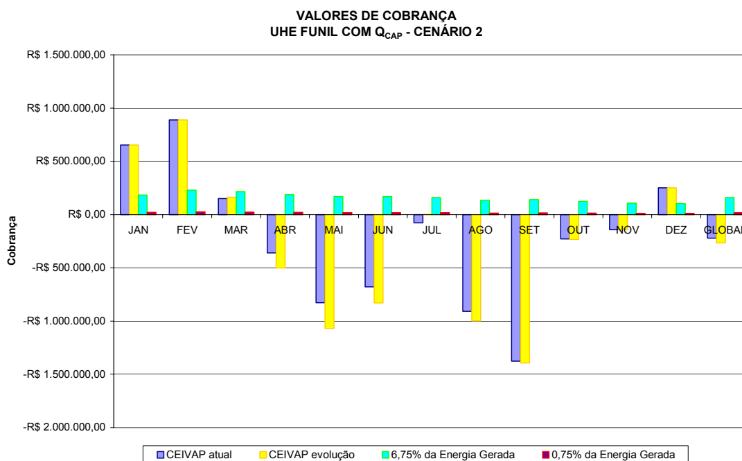
Figura 5.12 – Valores de cobrança simulados e atuais – UHE Funil – Cenário 2 com vazão de captação
