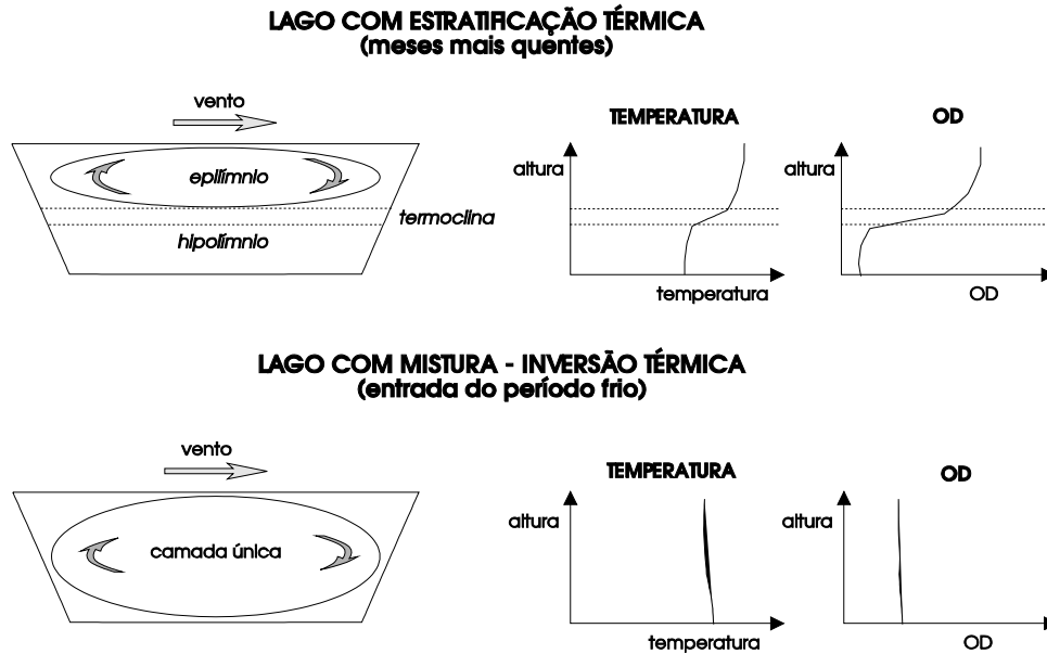
Figura 4.2 – Perfis de um lago em condições de estratificação e de inversão térmica (fonte: VON SPERLING, 1996)
