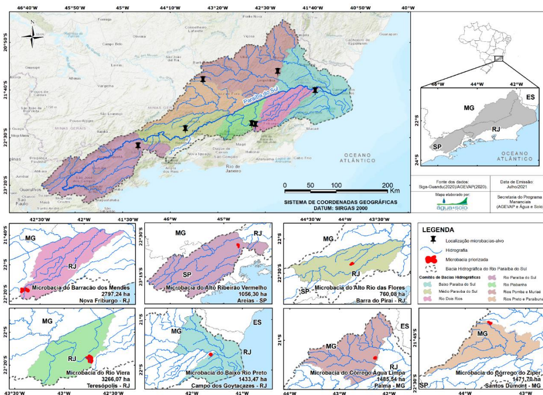
Figura 1. Localização das microbacias alvo do 1º ciclo do Programa Mananciais do CEIVAP.
